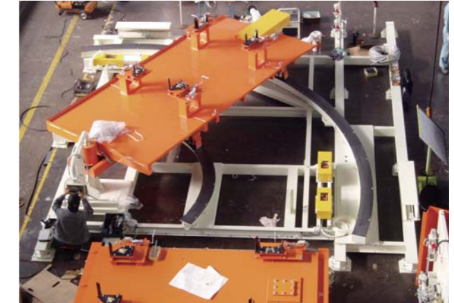
搬送治具付回転トラバーサ
