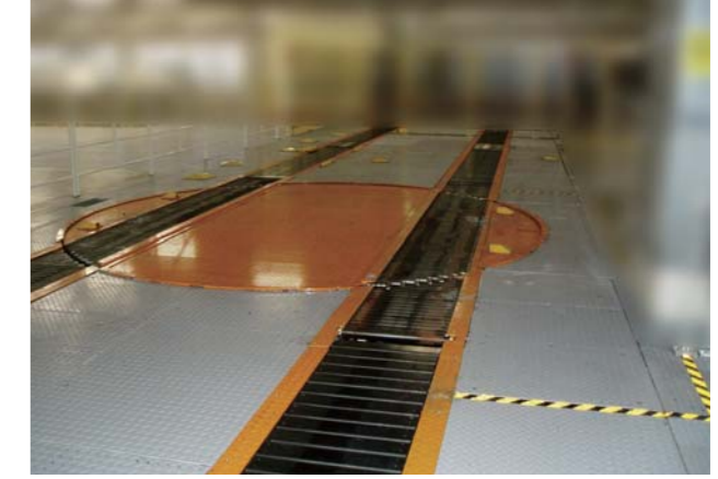
自動車ファイナルライン (スラットコンベヤ&ターンテーブル)
