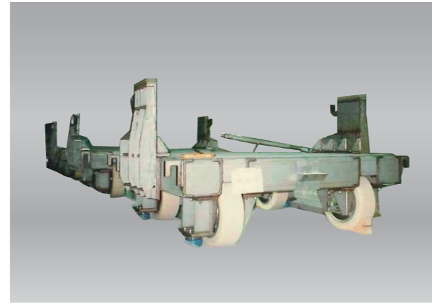
鉄道車両用仮台車
