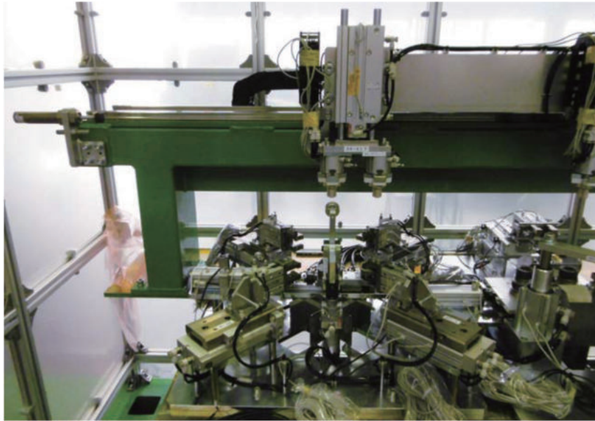
スプロケット自動組立ライン
