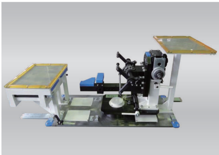
二輪車エンジン組立治具パレット 種類に合わせて治具の位置がスライド調整できます。
