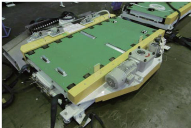
エンジン組立ライン(検査用、荷重1750kg、低床250H)
