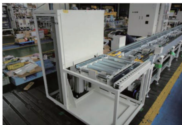
エンジン組立ライン (2層コンベヤ端末リフト、サイドプランジャ方式)
